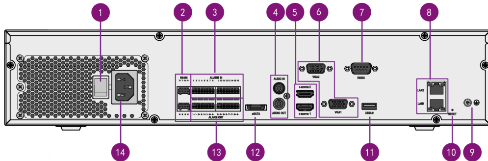
图 1-3 后面板示意图
