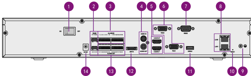
图 1-2 后面板示意图
