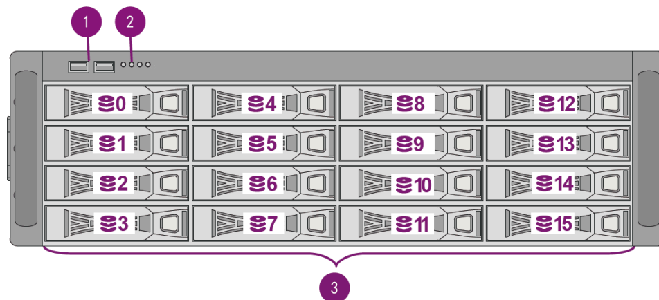
图 1-4 前面板示意图
